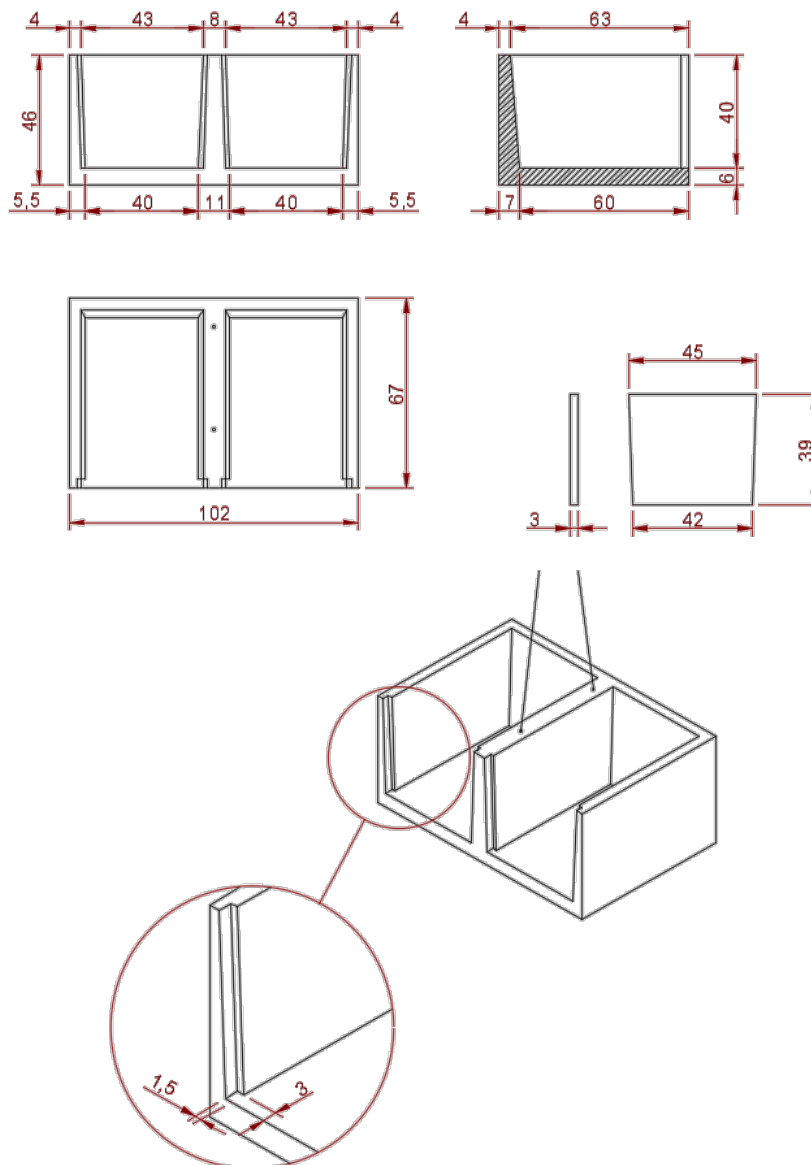
DETALLE A: REBAJE PARA ALQJAMIENTO DE LA TAPA FRONTAL
