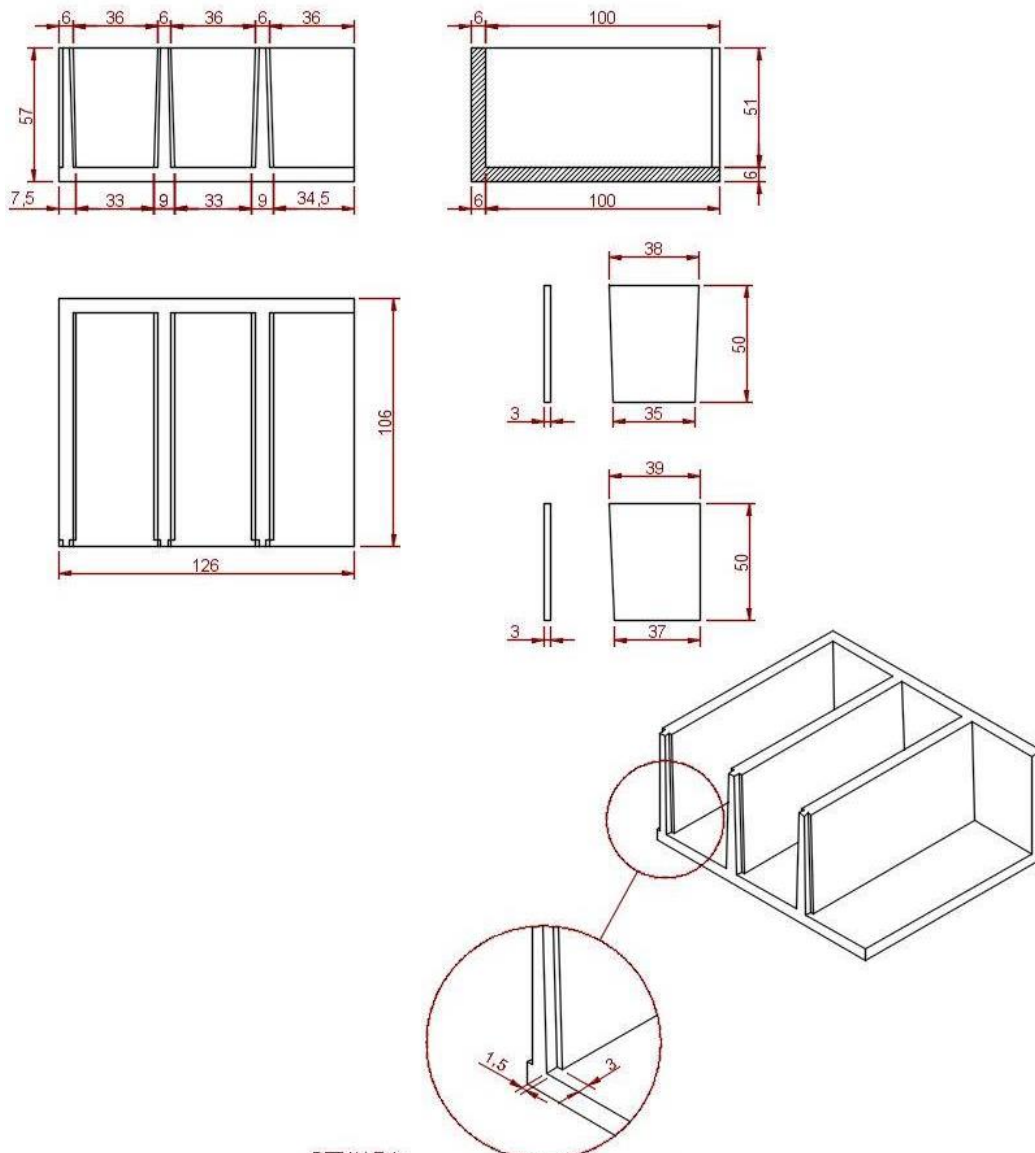
DETALLE A: REBAJE PARA ALOJAMIENTO DE LATAPAFRONTAL
